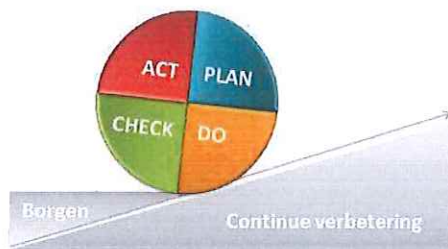
Fig. Cirkel van Deming
